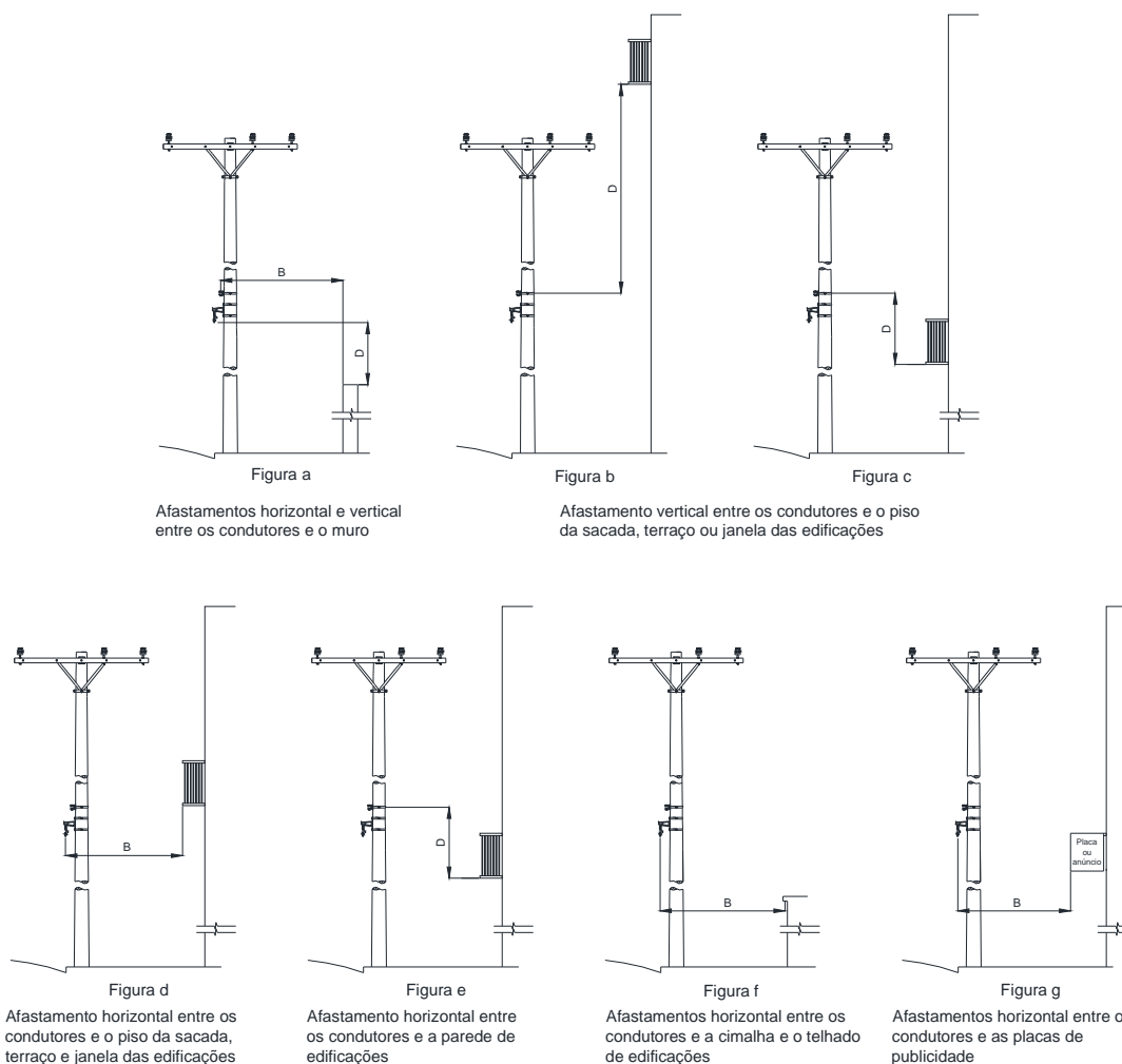
Figura 1 – Afastamentos mínimos – Condutores a edificações
