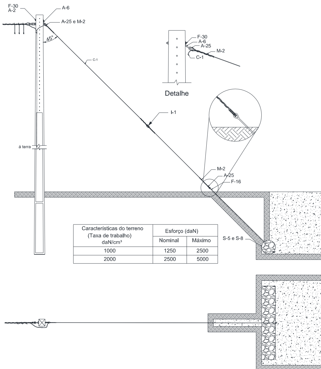
Figura 36 – Estaiamento – Estai de âncora
