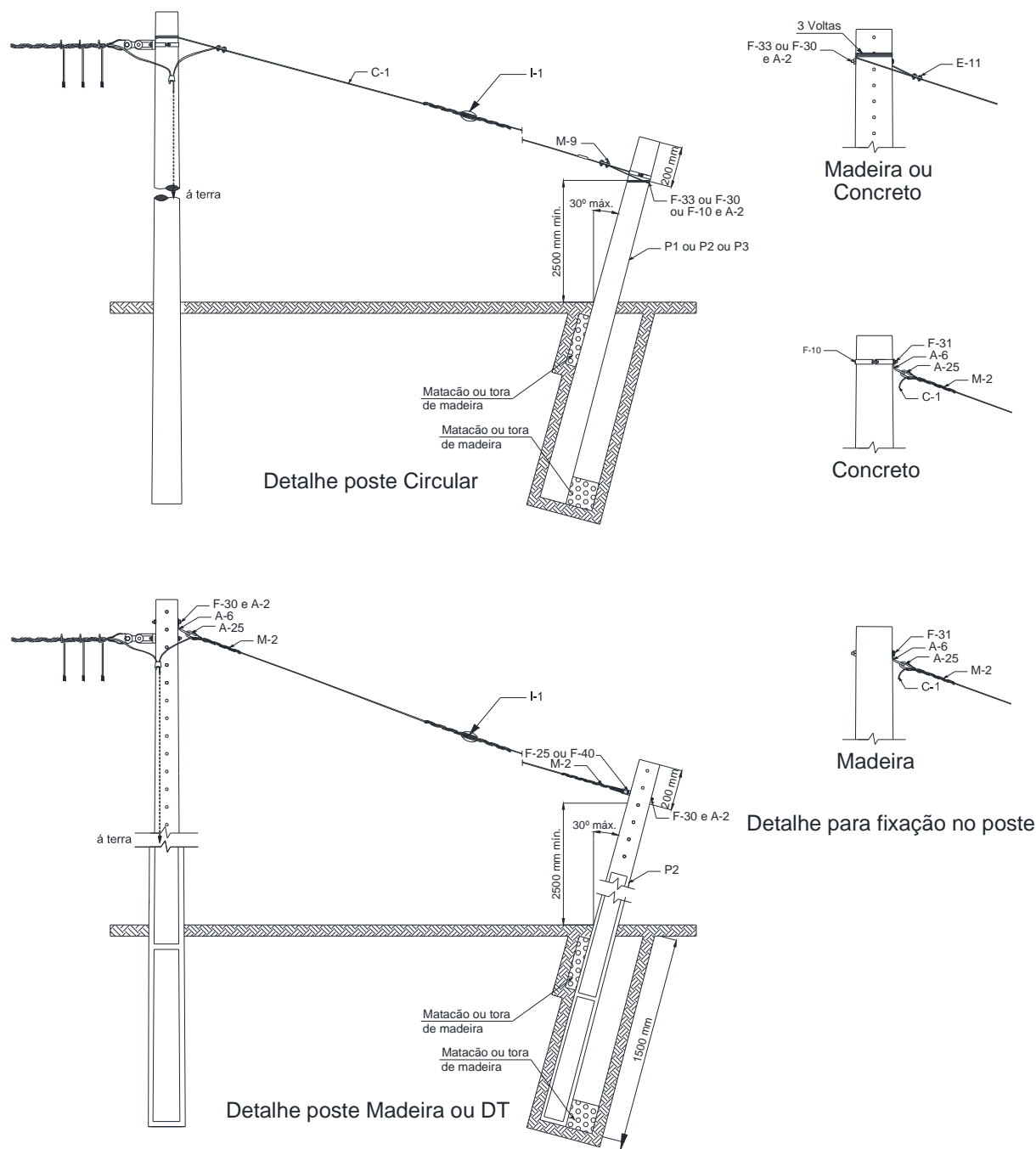
Figura 35 – Estaiamento – Estai com contra poste
