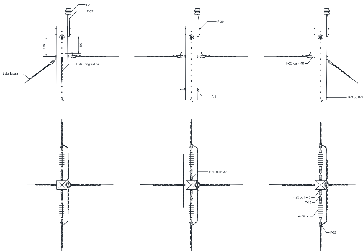
Figura 71 – Estrutura HTE – Poste de concreto de DT ou de madeira
