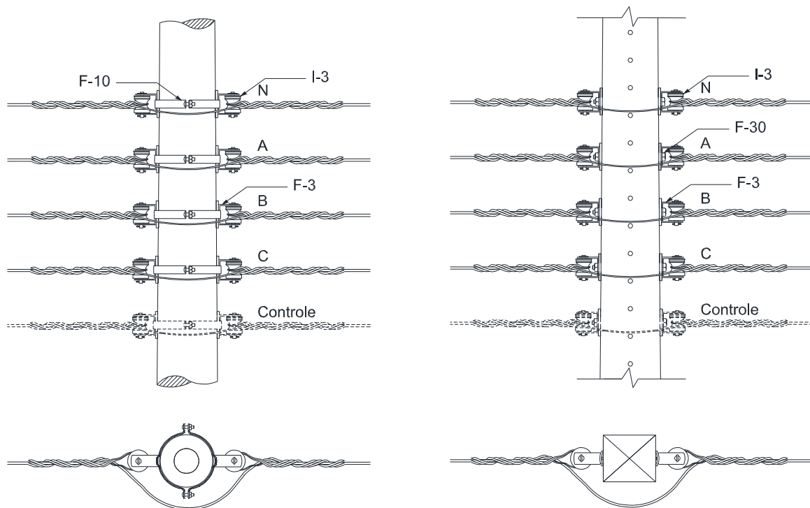
Figura 84 – Estrutura S4
