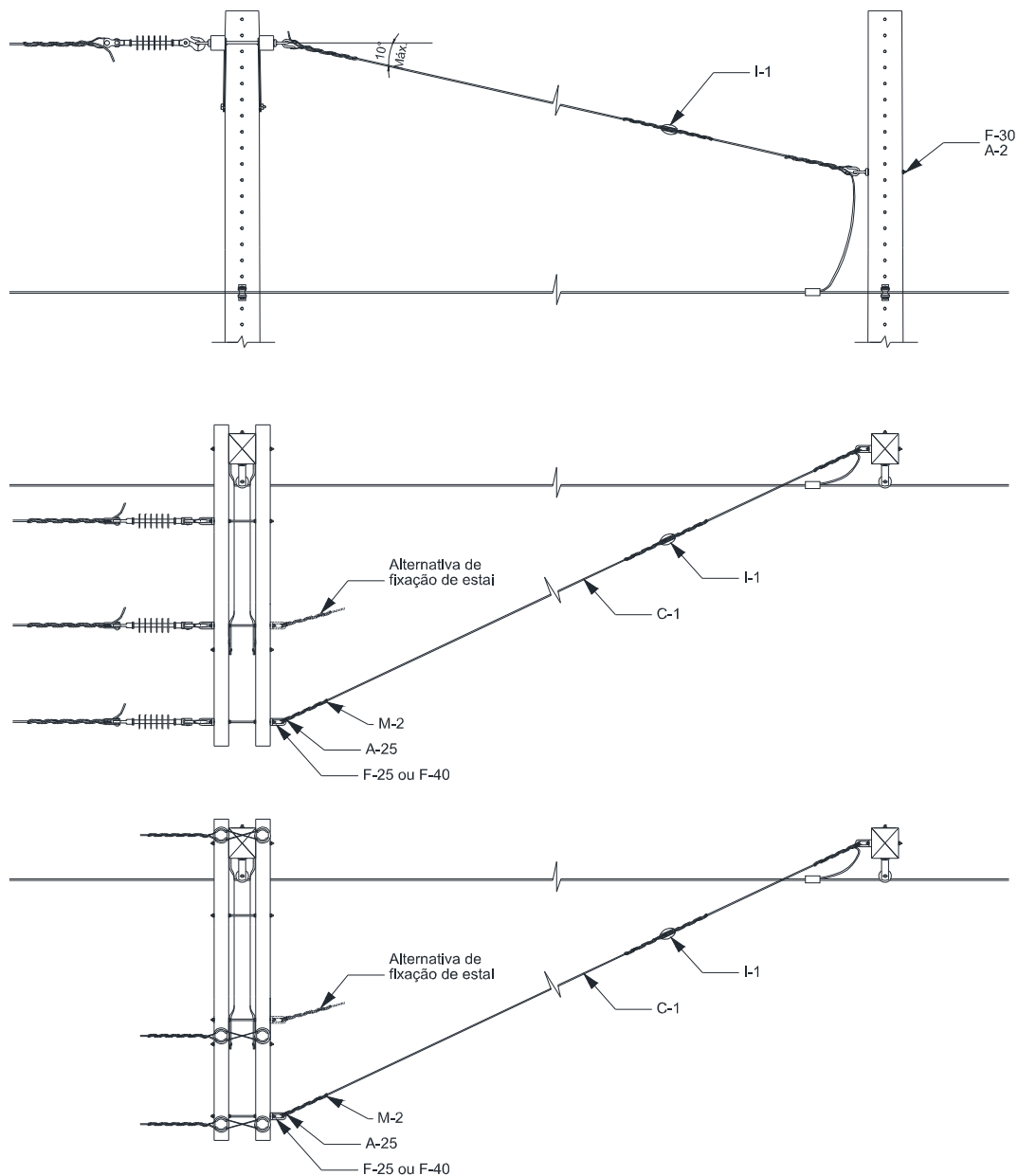
Figura 146 – Estaioamento – Estai de cruzeta a poste
