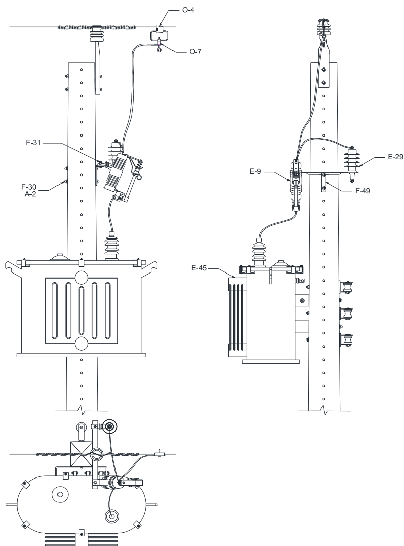
Figura 110 – Instalação de equipamento – Transformador monofásico – Estrutura monofásica
