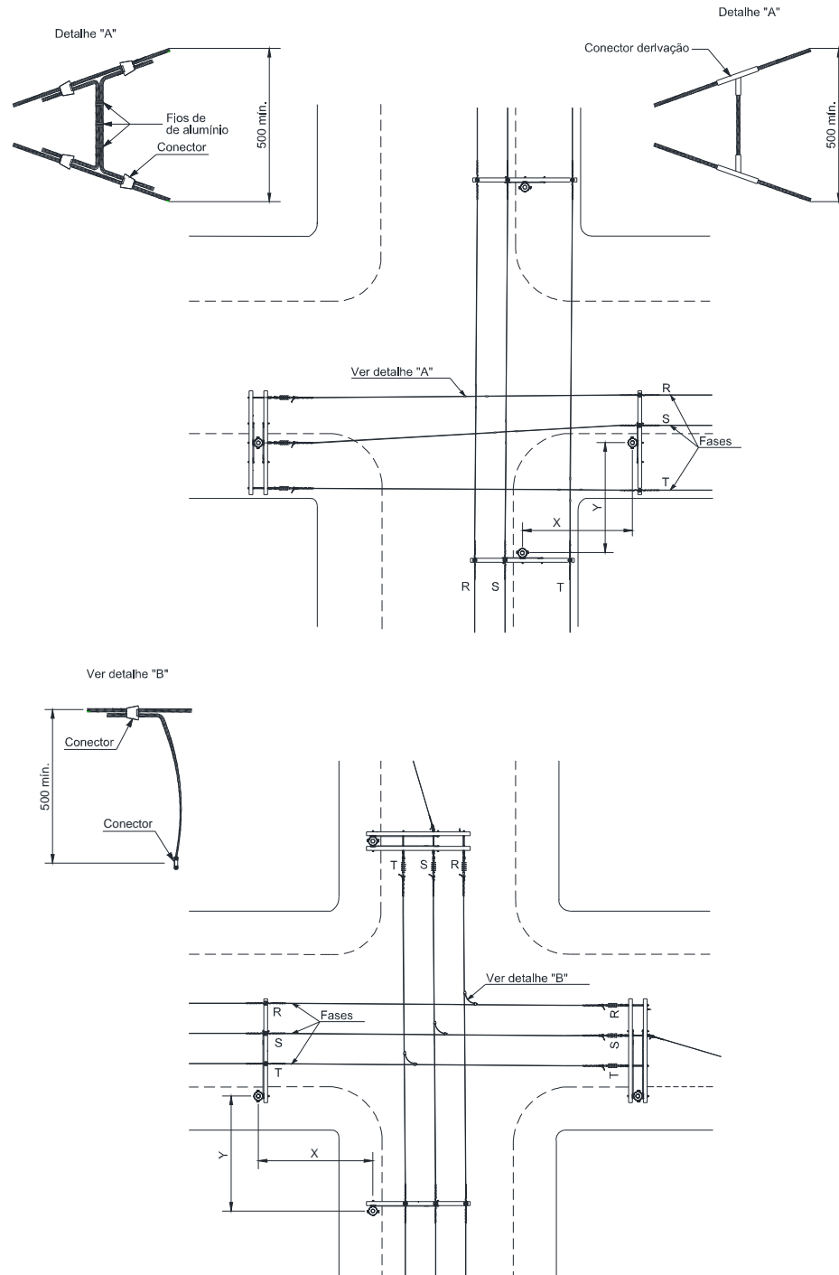
Figura 164 – Amarrações e ligações – Estrutura primária – Cruzamento aéreo
