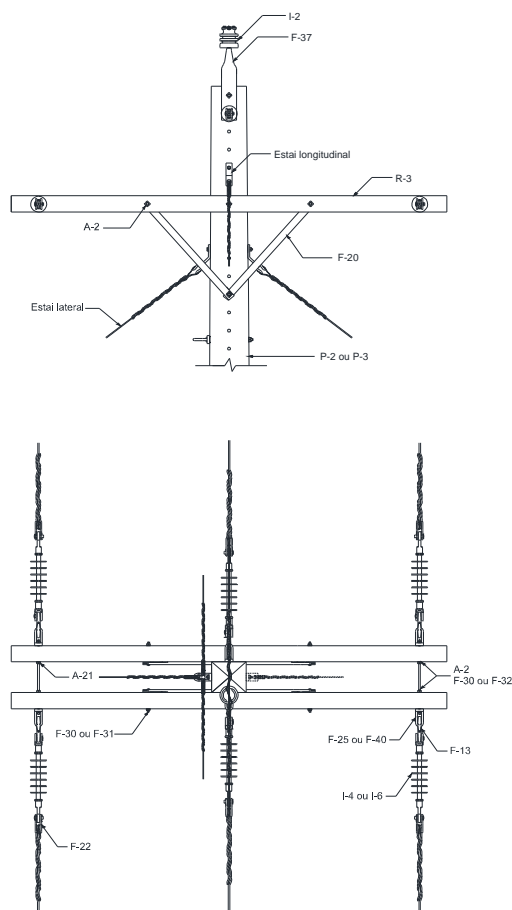
Figura 69 – Estrutura TE – Poste de concreto de DT ou de madeira
