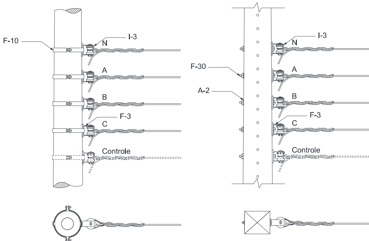
Figura 83 – Estrutura S3
